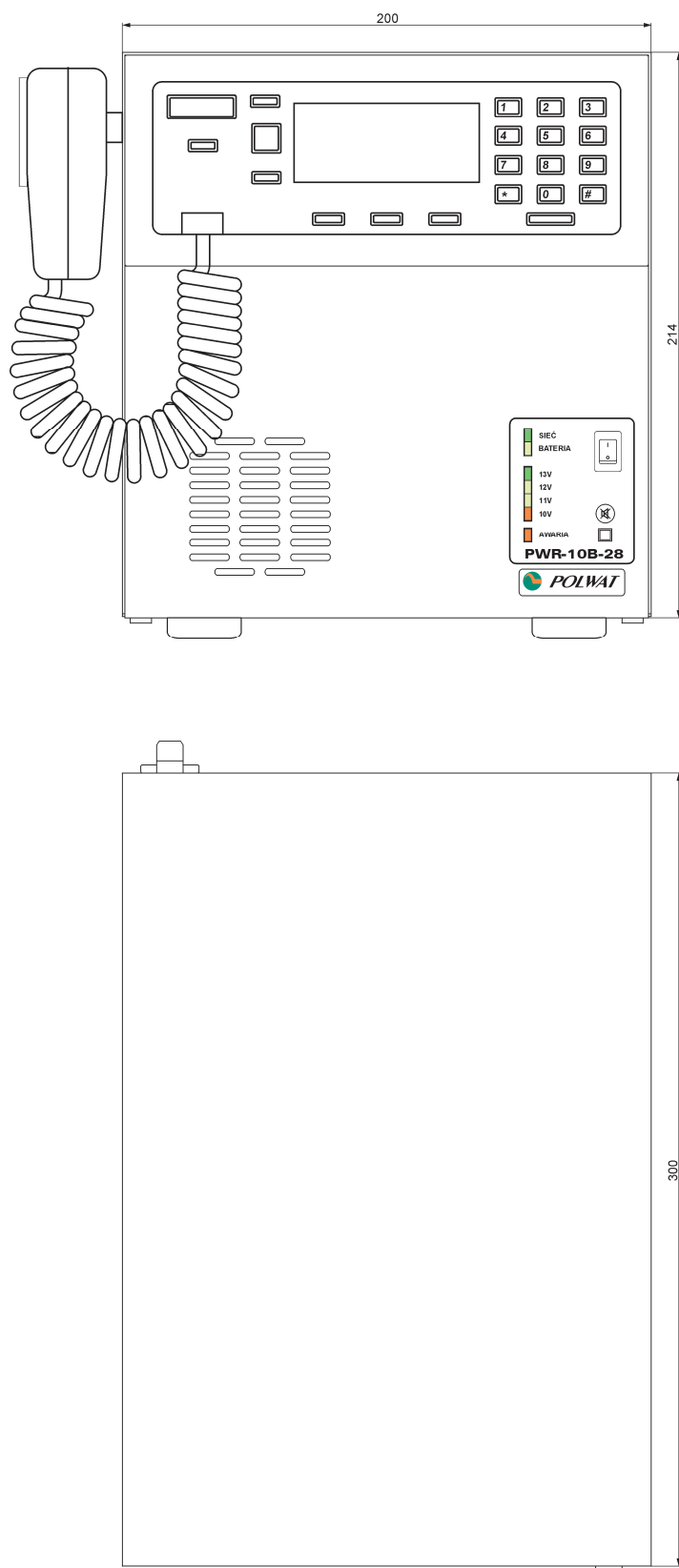
Rys.1. Wymiary gabarytowe zasilacza PWR-10B-28R
